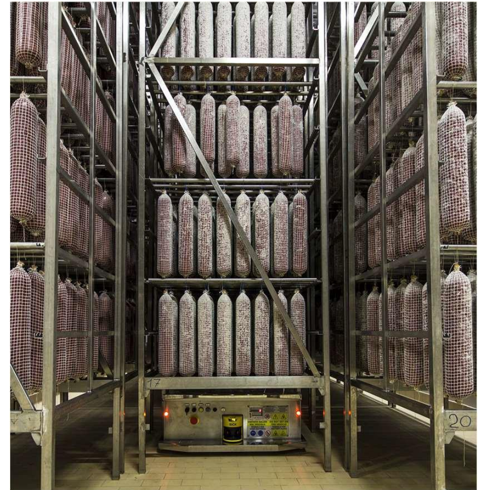
Shuttle in Edelstahlausführung mit eingebauten Wägezellen
